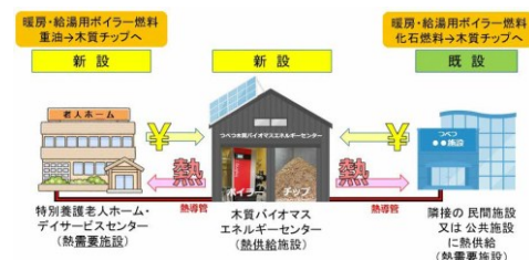
エネルギーの地産地消イメージ図
